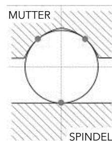
Funktion des profillosen Kugelgewindetriebs
